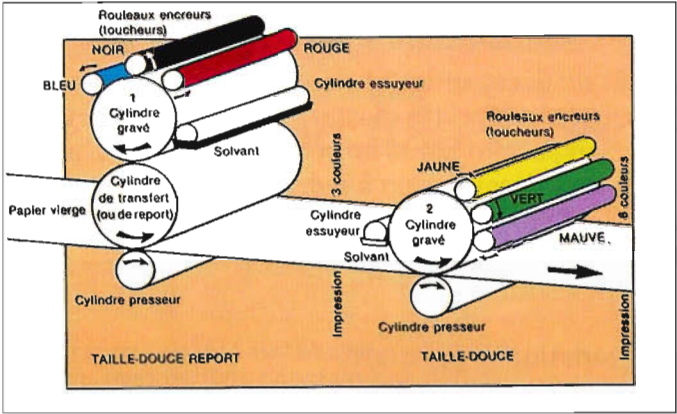
La taille-douce 6 couleurs (TD6). Deux cylindres d'impression appliquent chacun 3 couleurs justaposées sur le papier.
