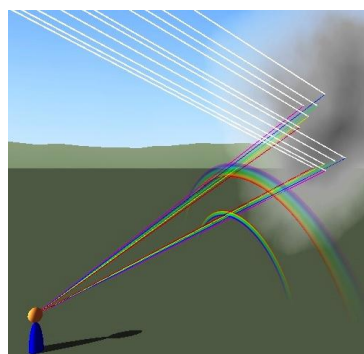
Schéma de principe de formation de l'arc-en-ciel.
