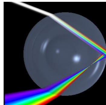
Réfraction et réflexion de la lumière dans une goutte d'eau.
