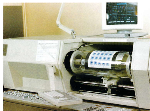
↑ Scanner rotatif.
